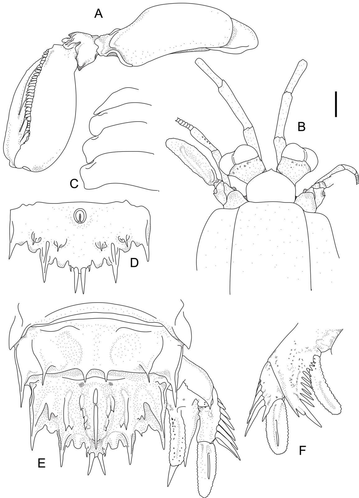
Fig. 3. Manningia australiensis Manning, 1970, ♂, TL 30 mm (IIOE2MOZ125). A. Left raptorial claw, lateral. B. Anterior cephalothorax, dorsal. C. TS5–8, left dorsal. D. Telson, ventral. E. Telson and left uropod, dorsal. F. Left uropod, ventral. Scale bar = 1 mm.
