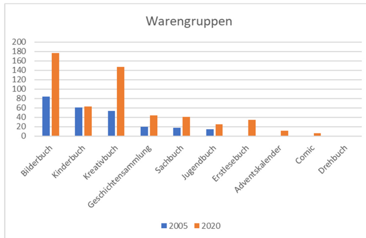
Abbildung 5: Warengruppen 2005/2020
