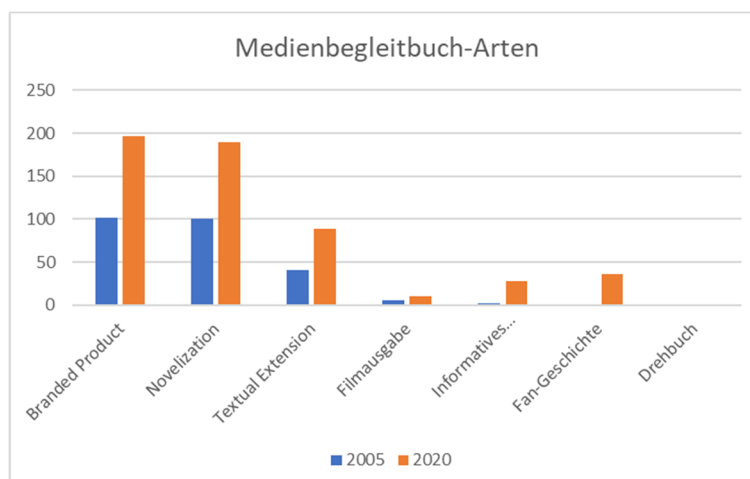
Abbildung 6: Medienbegleitbuch-Arten 2005/2020
