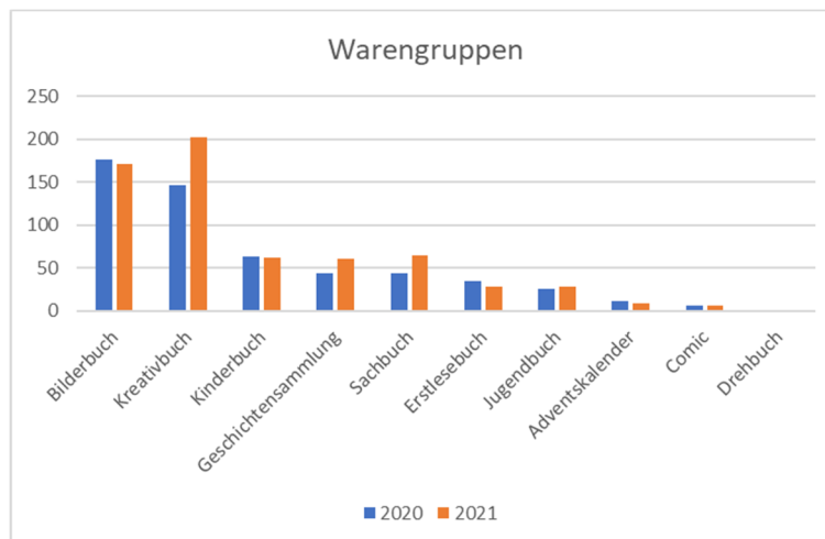
Abbildung 2: Warengruppen 2020/2021
