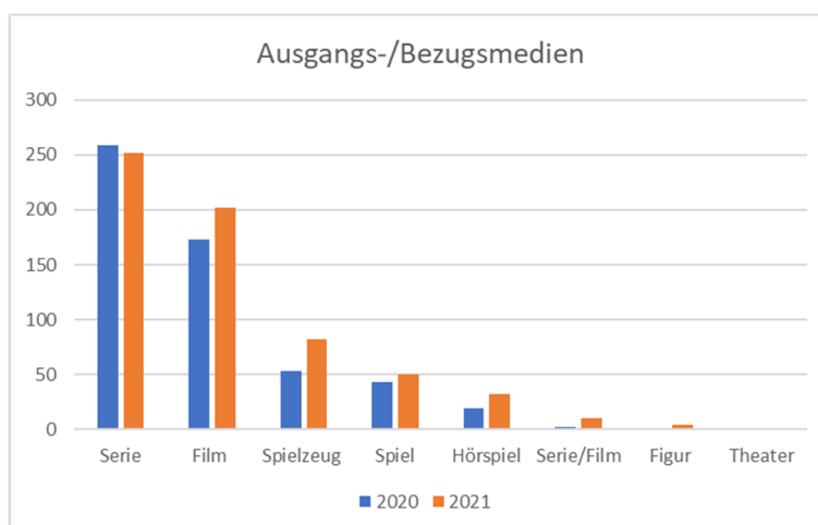
Abbildung 1: Ausgangs-/Bezugsmedien 2020/2021
