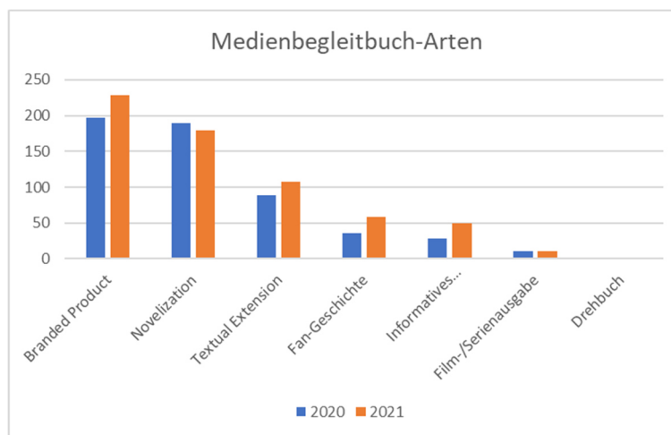
Abbildung 3: Medienbegleitbuch-Arten 2020/2021
