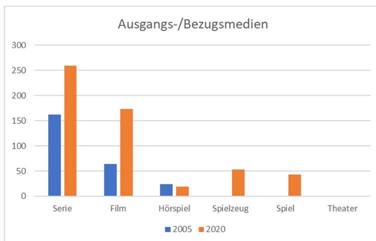
Abbildung 4: Ausgangs-/Bezugsmedien 2005/2020
