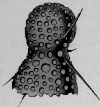
Fig. 20. Lithomelissa thoracites .
