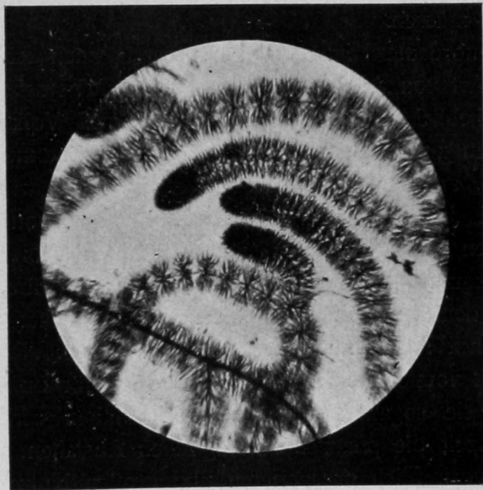
Fig. 25. Batrachospermum vagum .
