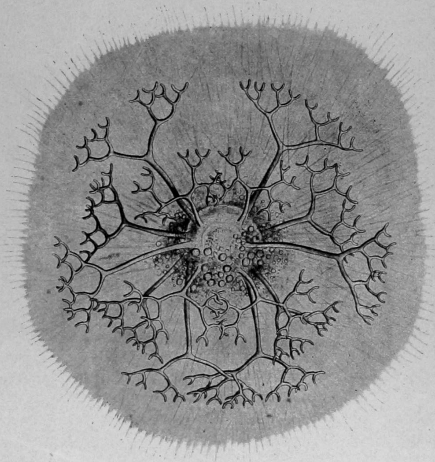
Fig. 18. Coclodendrum gracillimum .
