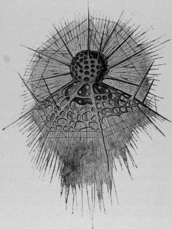
Fig. 19. Arachnocorys circumtexta .
