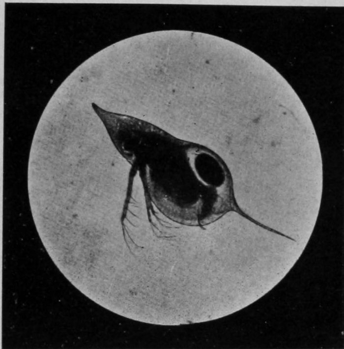
Fig. 21. Hyalodaphnia (Sommerform).
