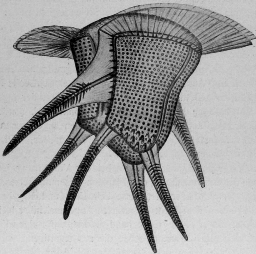
Fig. 13. Ceratocorys horrida .
