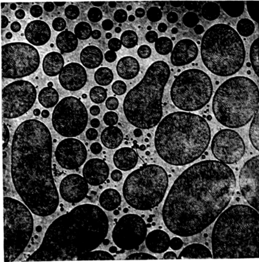
Fig. 8. Flüssige Mischkristalle,
