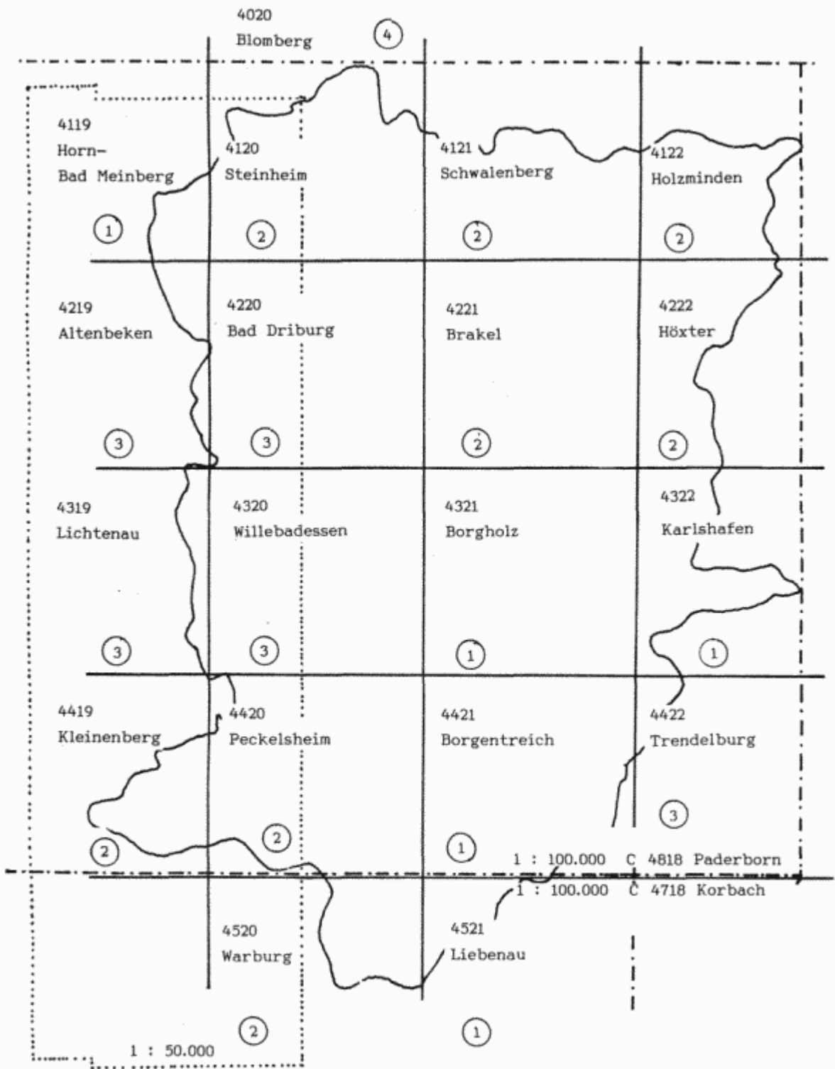
Abb. 1: — Geologische Karte: 1 : 25.000 ..... Geologische Karte: 1 : 50.000 - - - - Geologische Karte: 1 : 100.000
