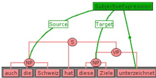
Figure 1: minimal tree covering auch die Schweiz hat diese Ziele unterzeichnet
