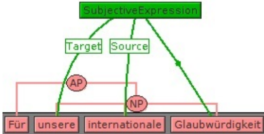
Figure 2: minimal tree covering Für unsere internationale Glaubwürdigkeit
